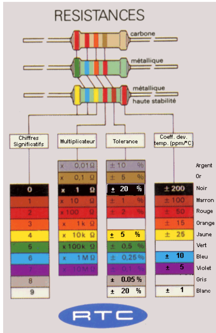
Code couleur des conducteurs ohmiques
